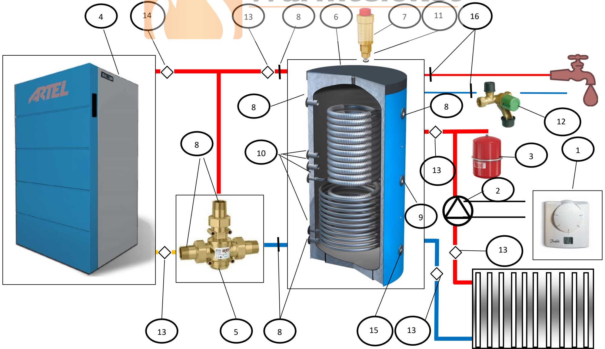
Aansluitschema Pelletketel in combinatie met hygiënebuffervat en warm tapwater
